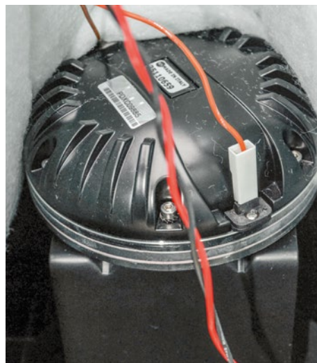
Driver o średnicy wylotu 1,5" to „kawał głośnika” – przetwornik wyposażony w neodymowy magnes, tytanową membranę oraz aluminiową cewkę o średnicy 4".
