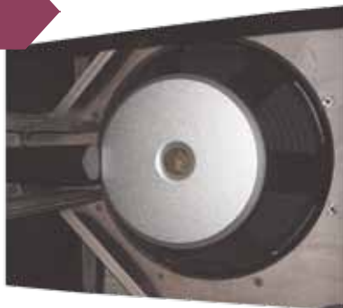
Głośnik 15" z zestawu szerokopasmowego wyposażono w tradycyjny ferrytowy obwód magnetyczny o średnicy 20 cm.
